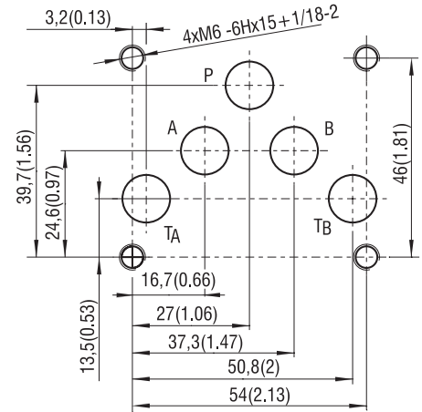
Dn 10 - ISO 4401-05-04-0-05
