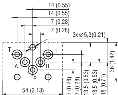
Dn 04 - CETOP-RP 121H
