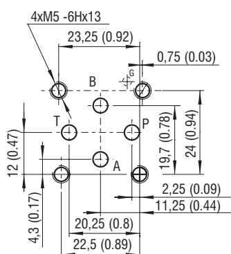
ISO 4401-02-01-0-05
