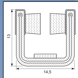
Rubber / fabric / brush 5 - 5,5 mm glass 40 x 0,3 mm steel
